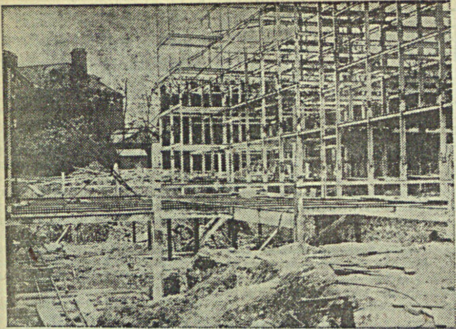
Строительство домов, защищенных против бомбардировки, в Англии. В гор. Ньюкестль (Англия) строятся жилые дома, защищенные против бомбардировки и снабженные газобезопасными. На снимке: вид строительства нового типа домов со стальными каркасами (Союзфото)
